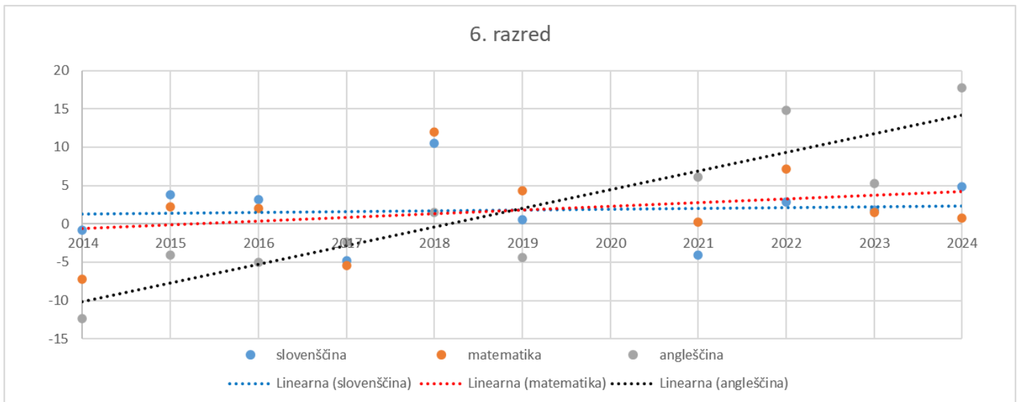
Graf 1: Trend rezultatov NPZ 6. razred od leta 2014 dalje.
