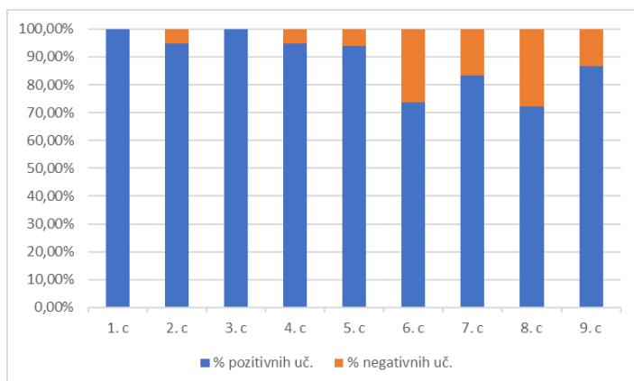
Graf 3: Prikaz % pozitivnih in negativnih učencev ob koncu pouka
