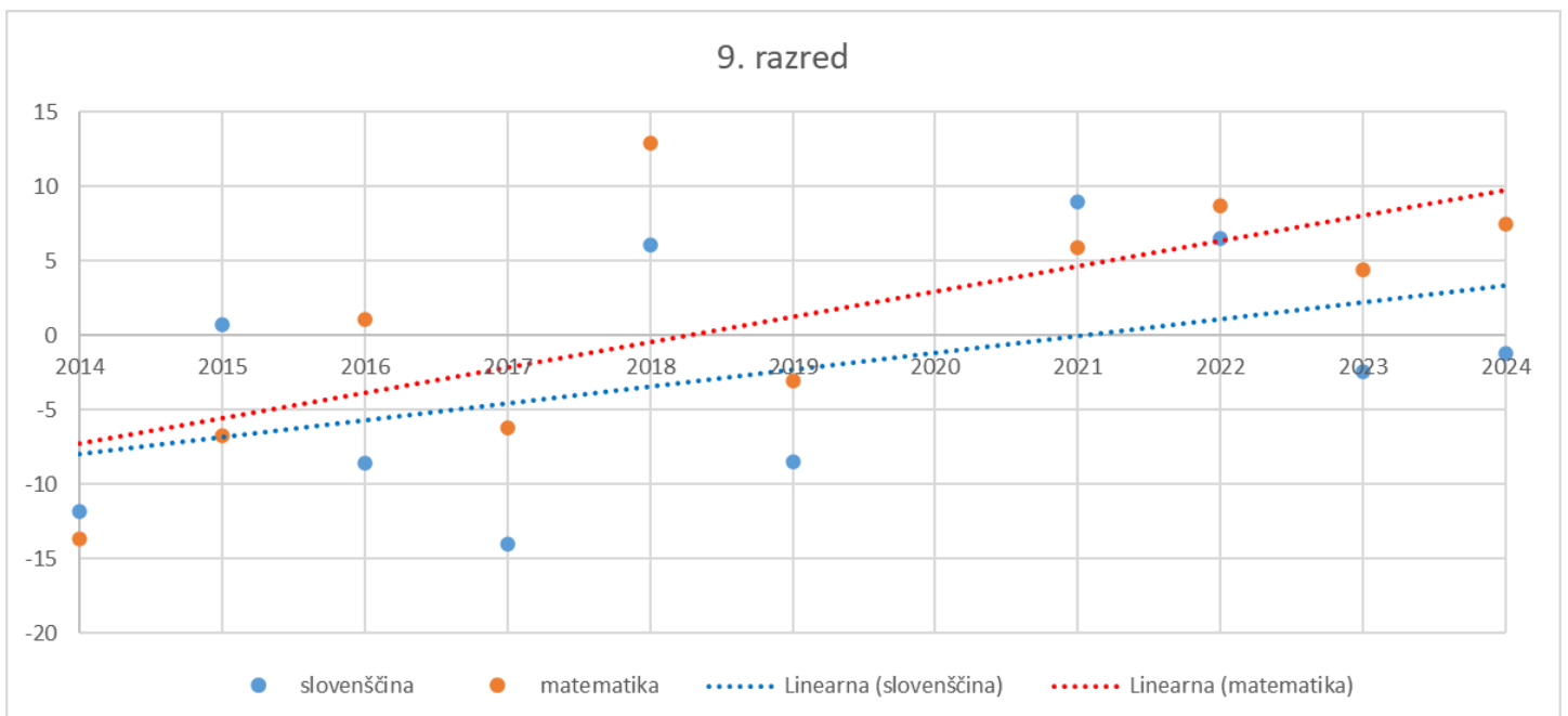
Graf 2: Trend rezultatov NPZ 9. razred od leta 2014 dalje.
